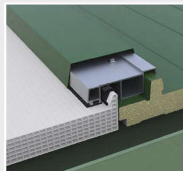
DETALLE LADO DERECHO Sistema completo con perfil-abrazadera
