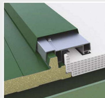
DETALLE LADO IZQUIERDO Sistema completo con perfil-abrazadera
