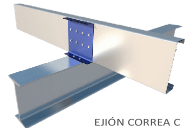
CUBREJUNTAS
