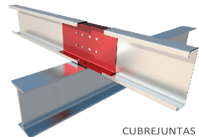
CUBREJUNTAS
