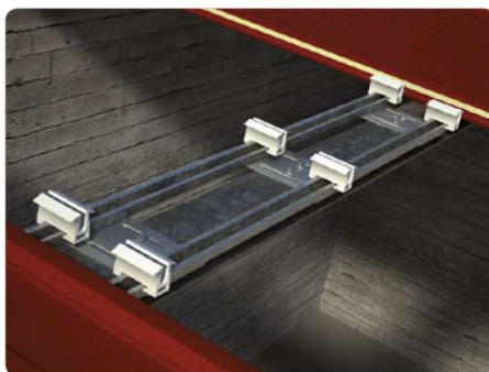
SOLAPE - 1ª FASE Detalle del soporte de enganche doble fijado en la estructura de cubierta
