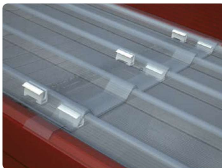
SOLAPE - 3ª FASE Colocación a presión de la placa superior
